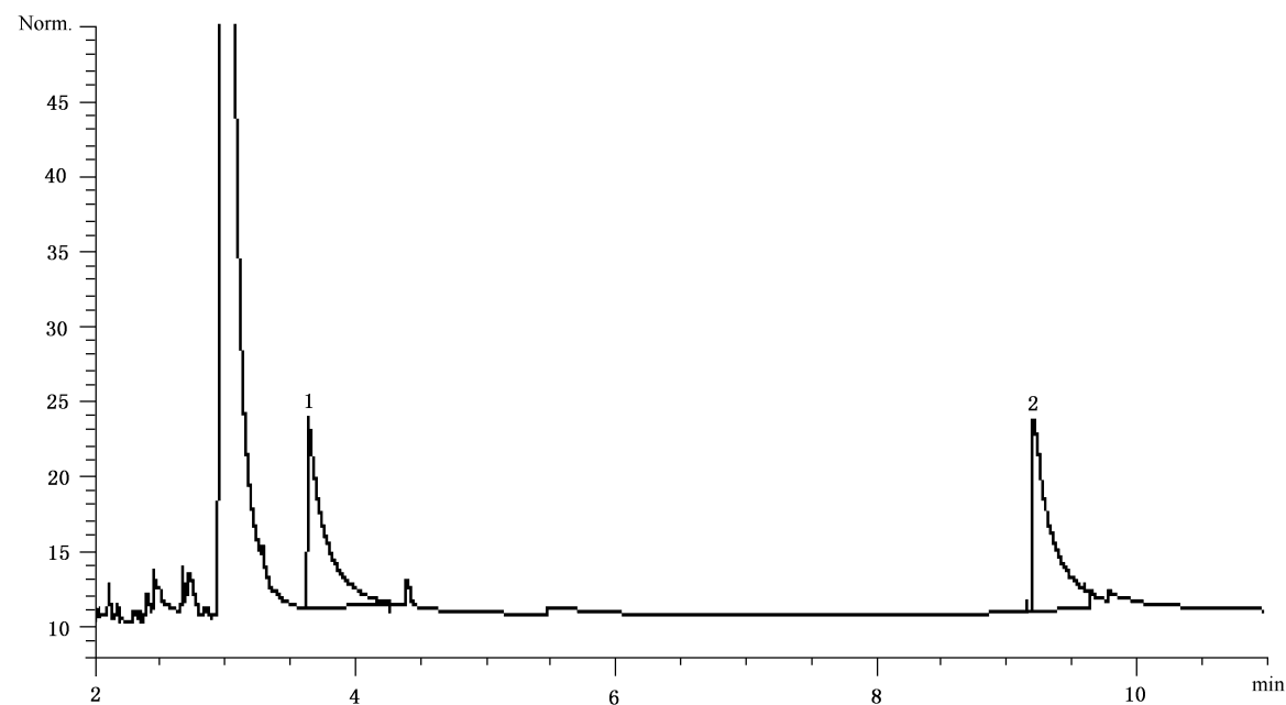
图 A.3 10%(体积分数)乙醇溶液中 2-( N,N -二甲基氨基)乙醇标准色谱图
